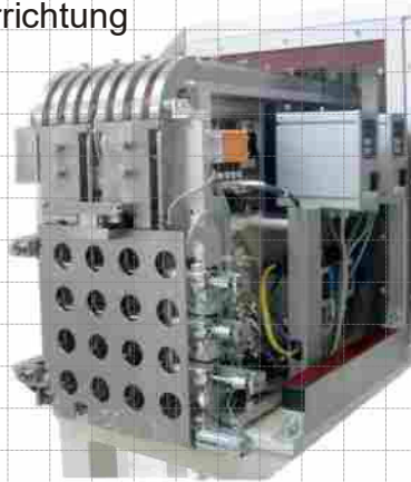
16-fach Ausstossvorrichtung
