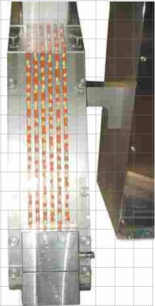
Zuführung 6-bahnig
