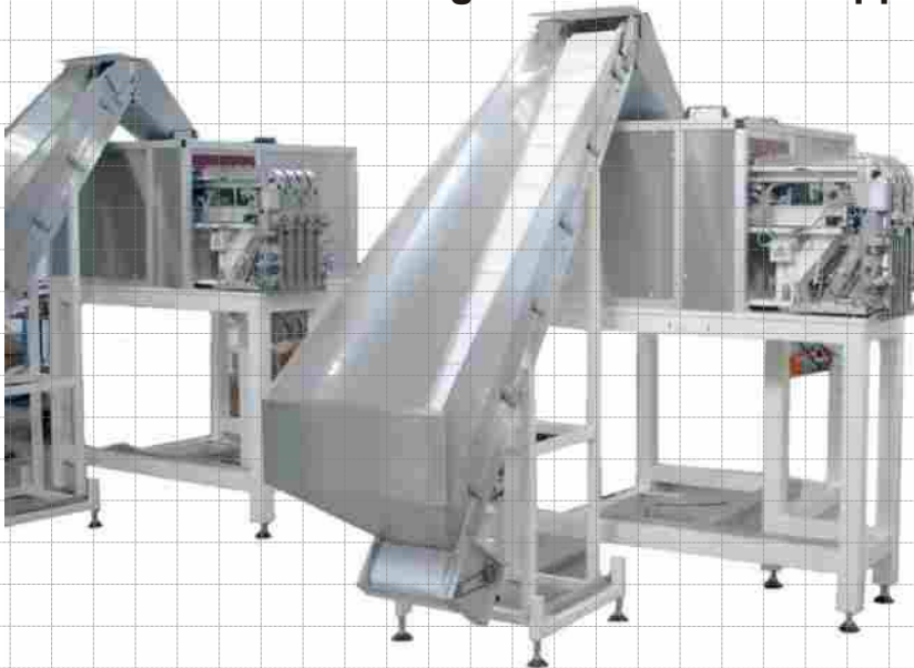
16-fach Ausstossvorrichtung
